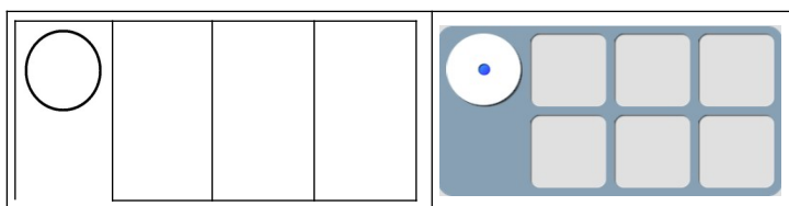
Шаблон 5.
