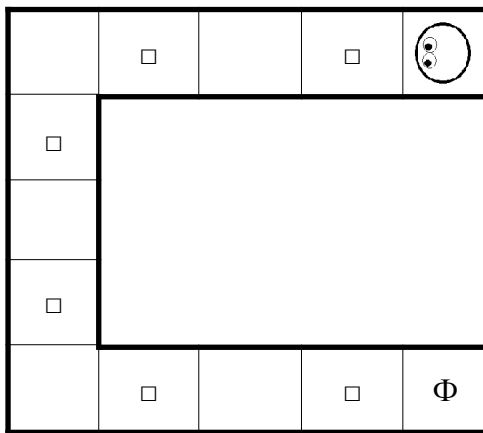
Шаблон программы:
