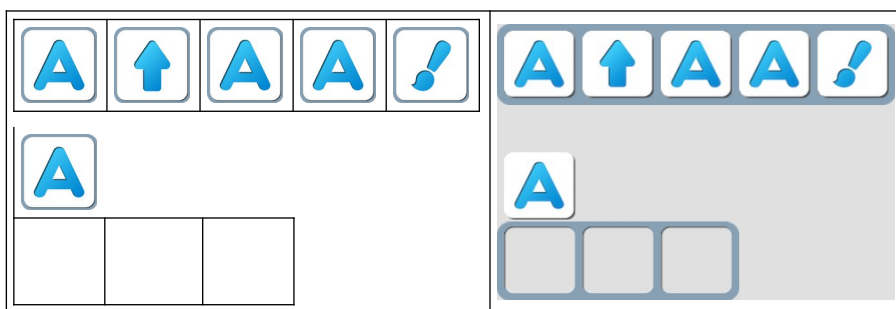
Шаблон 4.
