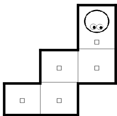
Шаблон программы:
